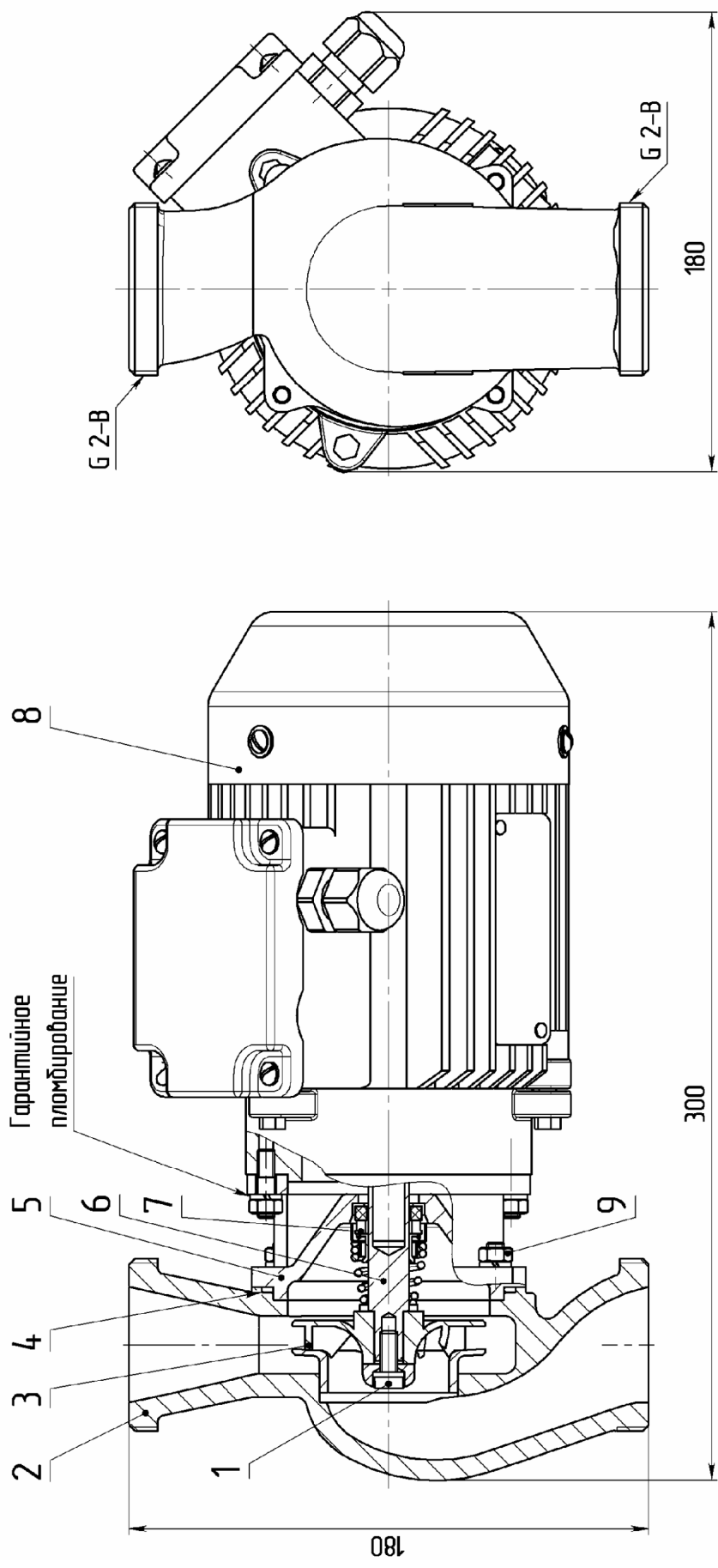
1— винт, 2 — корпус насоса, 3 — колесо насоса, 4 — кольцо, 5 — фонарь, 6 — муфта, 7 — уплотнение торцовое, 8 — двигатель, 9 — гайка М6.
